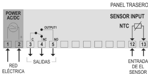
Figura 2 – Conexiones en el controlador (NTC)
