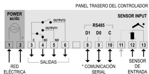
Figura 6 – Conexiones en el controlador
