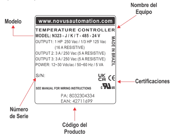
Figura 1 – Etiqueta de identificación
