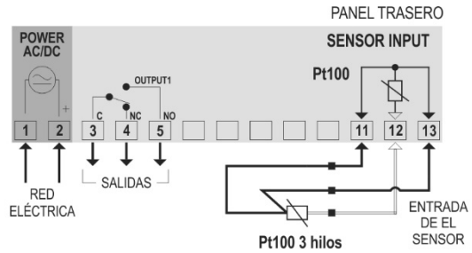
Figura 3 – Conexiones en el controlador (Pt100 3 hilos)
