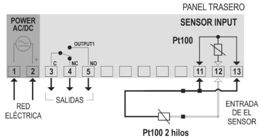
Figura 4 – Conexiones en el controlador (Pt100 2 hilos)
