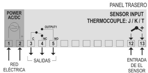
Figura 5 – Conexiones en el controlador (Termopar)
