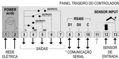
Figura 7 – Conexiones en el controlador
